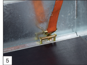
5 Standaard: bindbeugels geïntegreerd in de vloer: 1000 daN per stuk.
